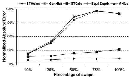
(a) Array \rightarrow Gauss .
