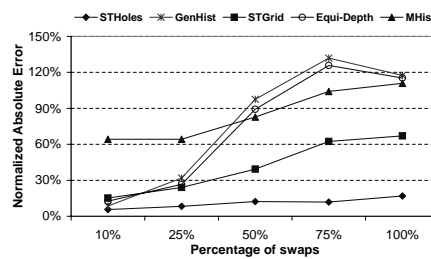
(b) Gauss \rightarrow Array .
